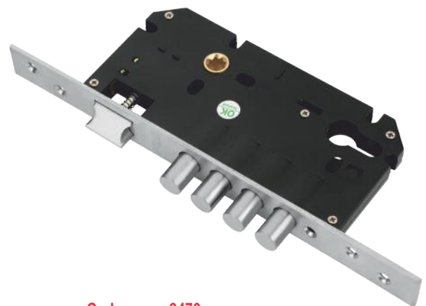
Code : 9470 Size : 9" (60mm x 85mm) Finish : SS, AB, CP
